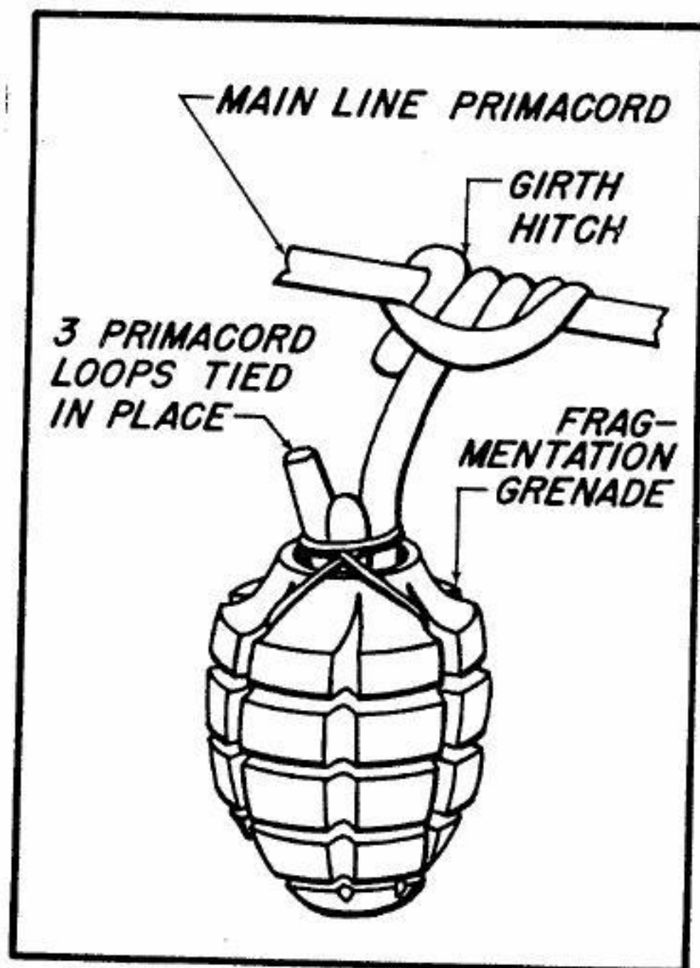
Fig. 46 — Frag Grenade Charge
